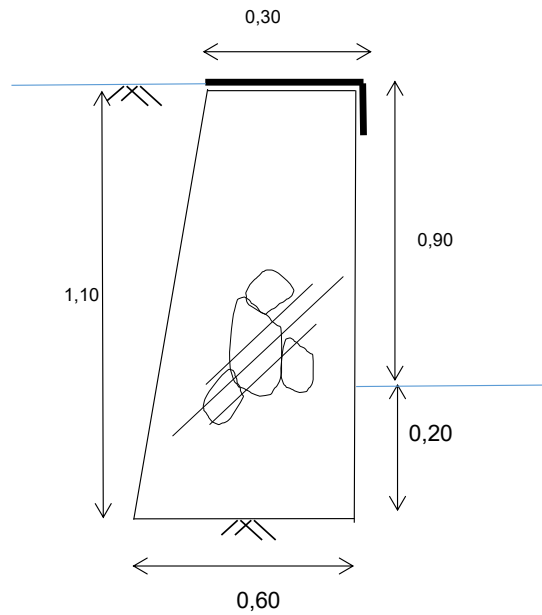
Potongan Melintang Talud Jalan
