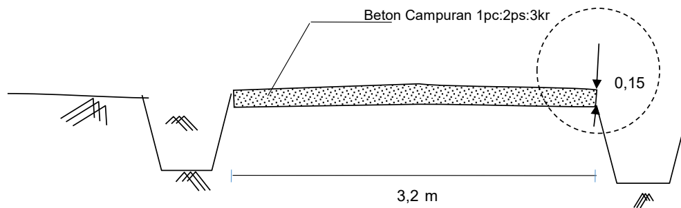
POTONGAN MELINTANG
