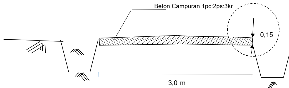
POTONGAN MELINTANG
