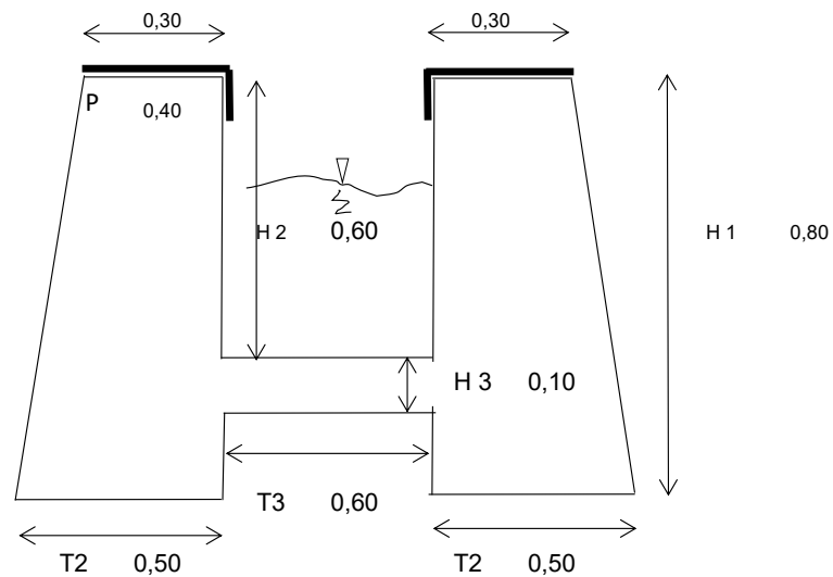
Potongan Melintang
