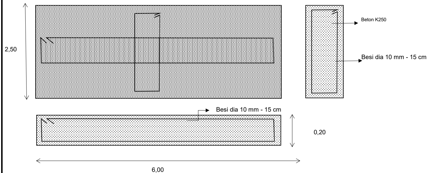
Gambar Plat Beton Tanpa skala
