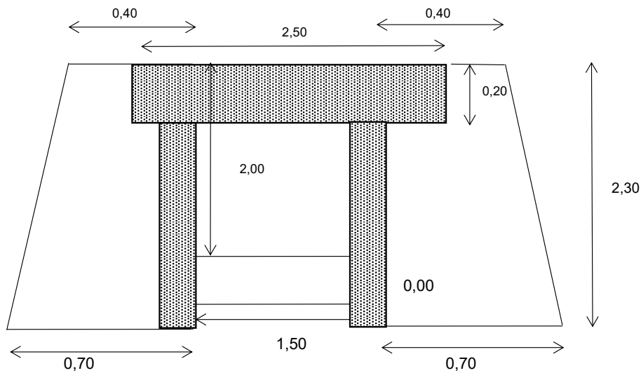
Potongan Melintang Gorong-Gorong Plat Tanpa skala
